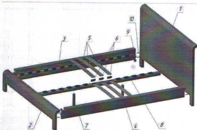
Рис.1 Сборка кровати
