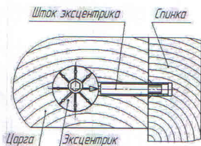
Рис.2 Стяжка эксцентриком
